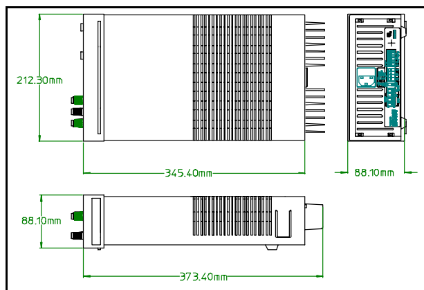
Abbildung 1. Maßskizze
