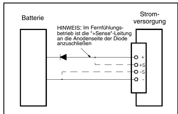
Abbildung 17. Empfohlene Schutzschaltung für das Laden von Batterien
